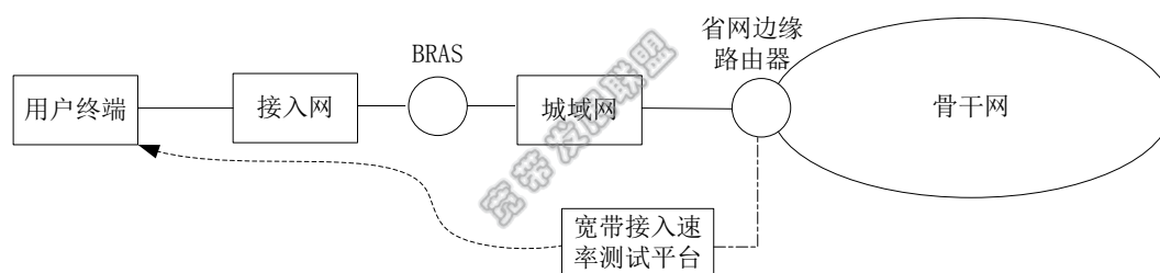
图 18 第二替代测试方法连接图
