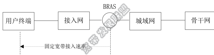
图 17 固定宽带接入对应的网络位置
