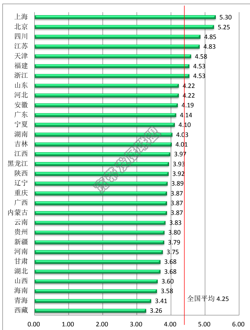
图5 各省忙闲时加权平均可用下载速率（单位：Mbit/s）
