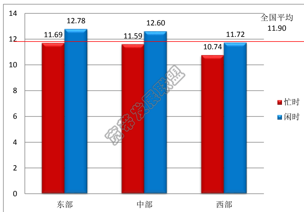
图4 忙、闲时平均可用下载速率区域对比（单位：Mbit/s）
