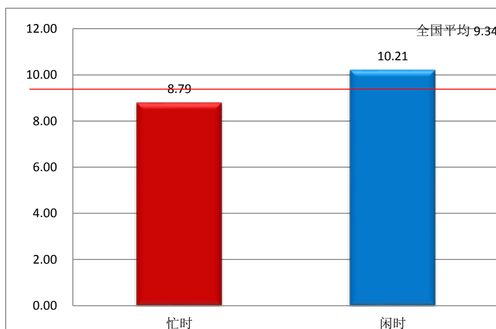
图12 全国平均视频下载速率忙、闲时对比（单位：Mbit/s）
